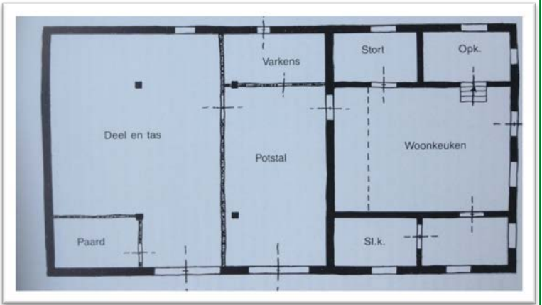
Plattegrond groot hallehuis (Thijs Pubben)
