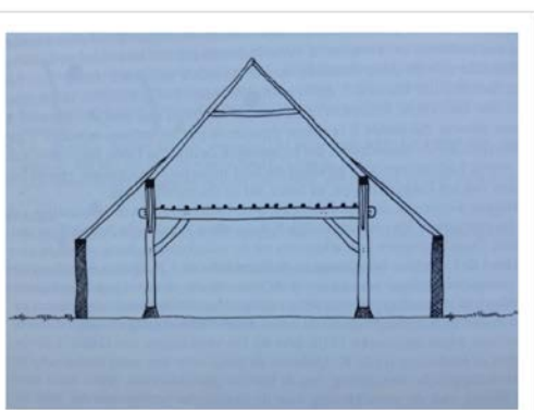
Gebint met sporenkap (Thijs Pubben)
