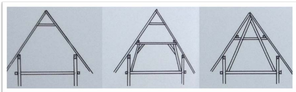
Kapconstructies voor een hallehuis sporenkap
