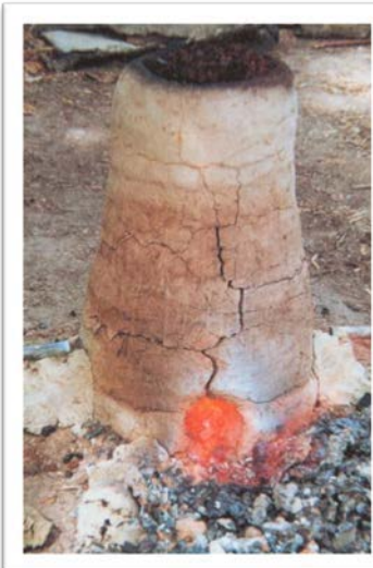
Schachtoven (Leo Verhart)
